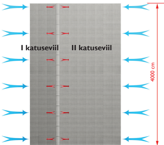
Joonis 12. Üks plaatide nurkade lõikamise näide. Lõige on tehtud betoonilõikekettaga varustatud nurklihvijaga. oonised – katuse projektsoon ja läbilõige – on esitatud tuulutusavade arvutamise näidisenä. Sinised nooled tähendavad õhu sissepääsuavasid, punased nooled aga õhu väljapääsuavasid katuseharja juures.
