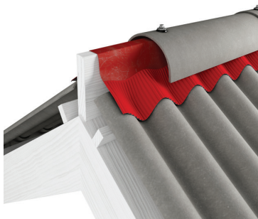
Joonis 7. Harjadetaili ja tihendusribaga kaetud katuseharja: tuulutusavade pindala katuseharja 1 jooksva meetri kohta: plaadid W130-9 – 150 cm 2 iga katuseviilu kohta.
