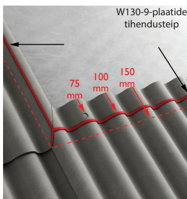
Joonis 19. Risti- ja pikisuunaliste ülekattete tihendamine teibigakatuseviilu kalde korral 22° (40 protsenti).
