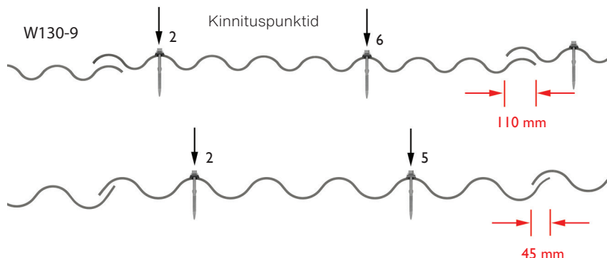
Joonis 24a. Plaatide W130-9 kinnituspunktid on 2. ja 6. laine harjal. Siin on kujutatud katusevillu katmist vasakult paremale.
