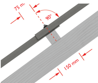
Joonis 18. Plaadid W130-9 paigaldatakse 150 mm ülekatttega. Kinnituskrui keeratakse roovilatti otse risti.
