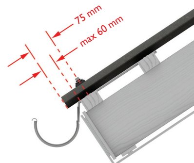
Joonis 20. Kaugus kinnituspunktist plaadi alumise servani on 75 mm.
