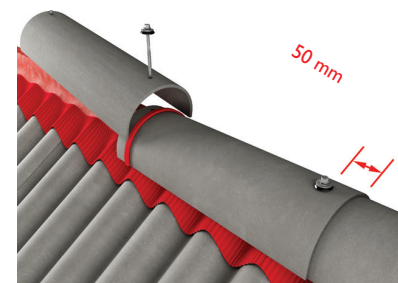
Joonis 35. Poolsilindri kujulise harjadetaili paigaldamine.
